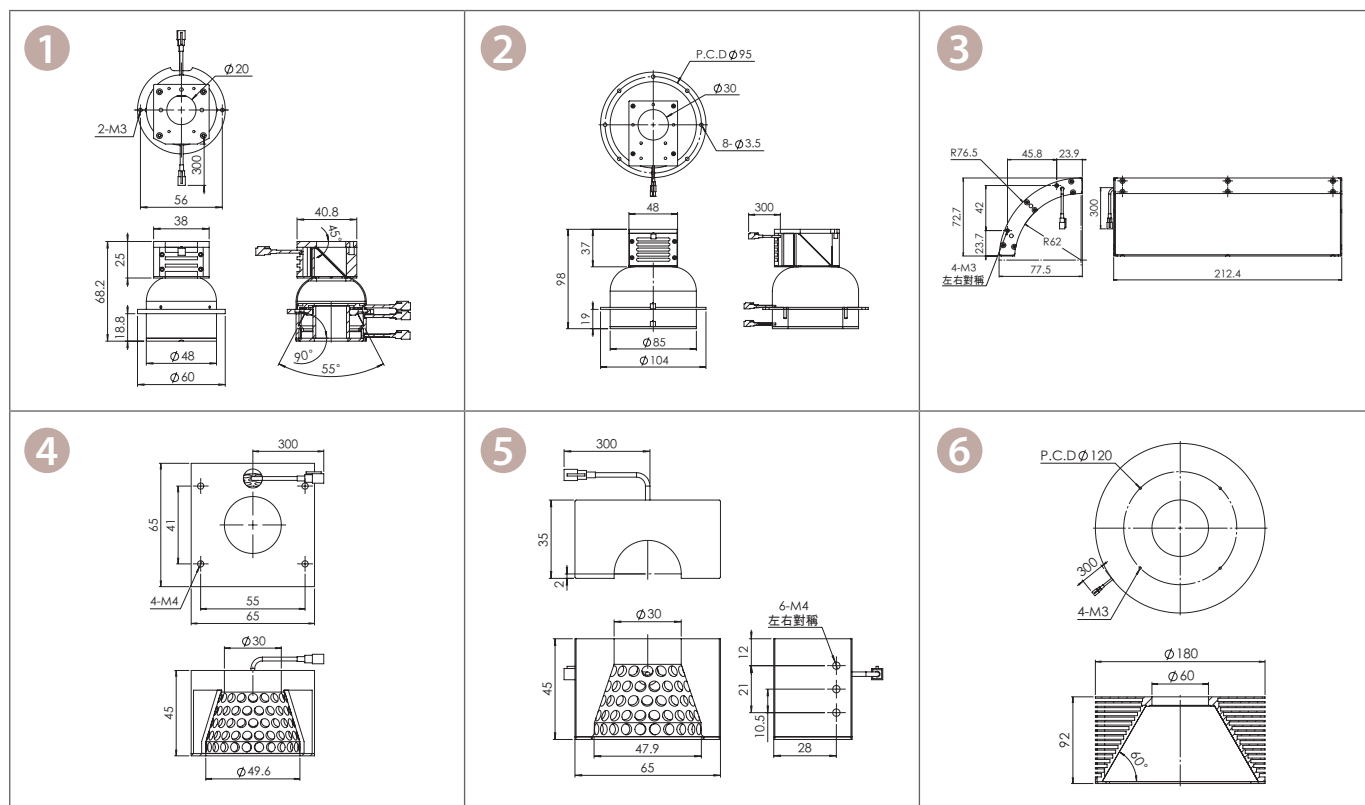
■ 尺寸圖 Dimension (mm)
