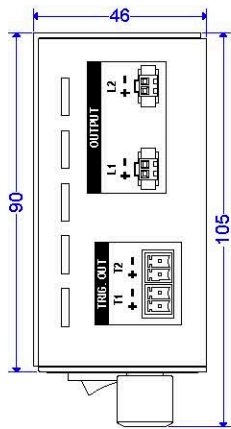
上視圖
