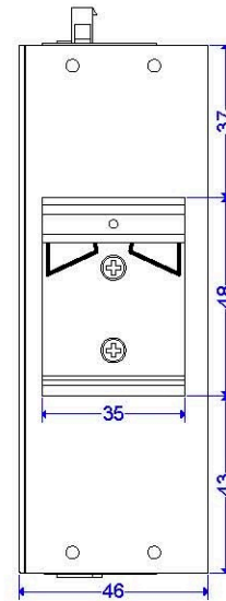
導軌卡扣
