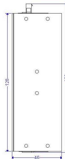
後視圖
