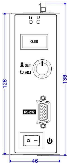
前視圖
