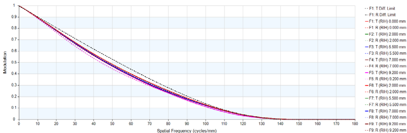
全頻 MTF F#14
