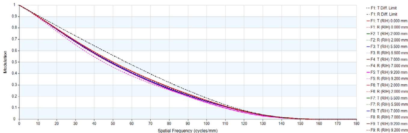
全頻 MTF F#13
