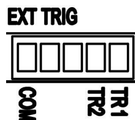
圖 3 外觸發輸入介面
