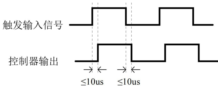
圖7 常減模式時序圖
