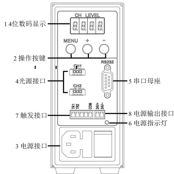
圖 1 前面板
